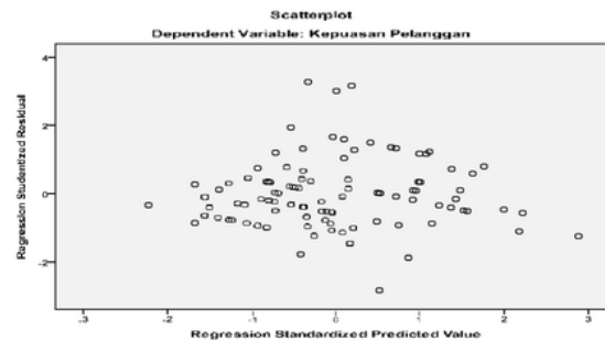
Gambar 2. Grafik Scatterplot Uji Heterokedastisitas
